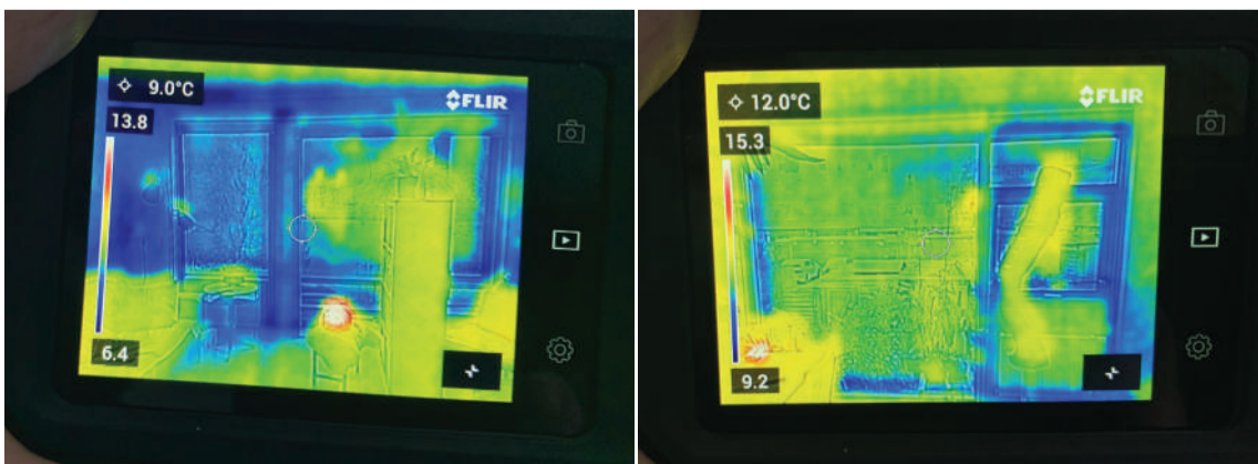
Warmtescan van de ramen van de woonkamer aan voor- en achterkant. De kleuren geven aan waar warmte verloren gaat (blauw is koud).
